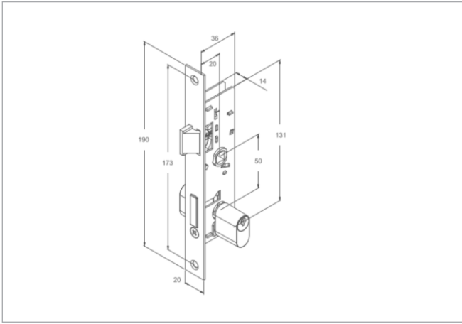
Código Descrição - *medidas em mm 224 FECHADURA STAM 602 ESTREITA
