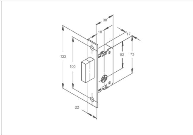
Código Descrição - *medidas em mm 246 FECHADURA SEGUR STAM PAR 1003
