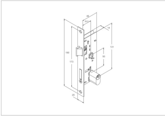
Código Descrição - *medidas em mm 225 FECHADURA STAM 502 MÉDIA
