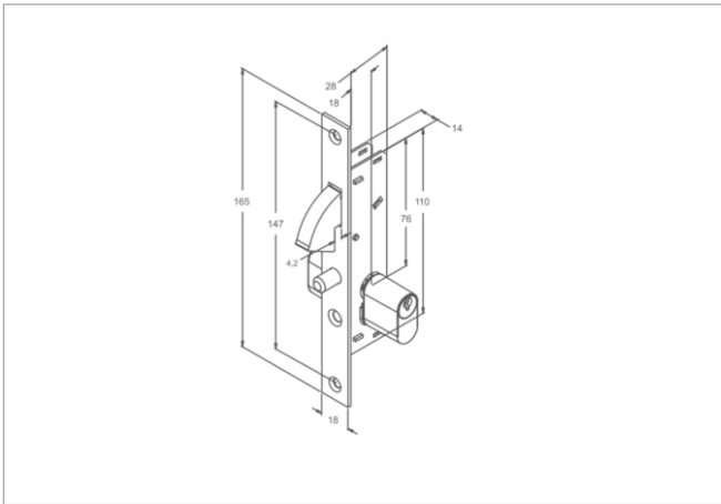
Código Descrição - *medidas em mm 226 FECHADURA STAM 901 BICO DE PAPAGAIO
