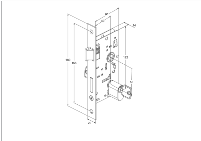
Código Descrição - *medidas em mm 1904 FECHADURA STAM 803 LARGA
