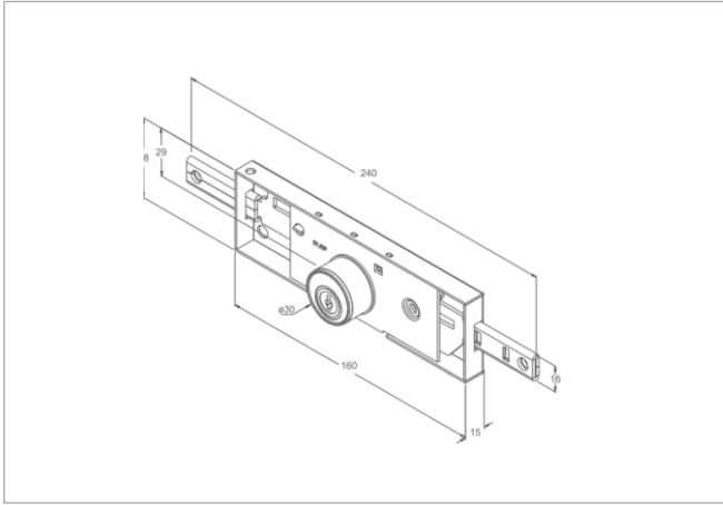
Código Descrição - *medidas em mm 227 FECHADURA STAM 201 PORTA DE ENROLAR
